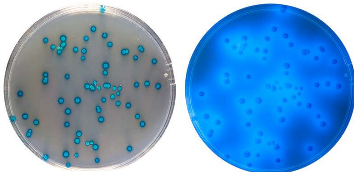
A sinistra: colonie di E. coli alla luce naturale; a destra: la stessa piastra sotto lampada di Wood
