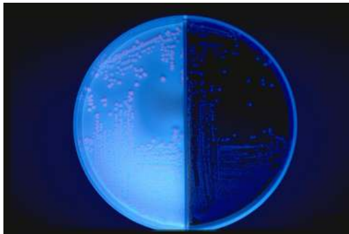
Biosector 3 alla lampada di Wood: colonie di E. coli , fluorescenti su Mac Conkey Agar MUG
